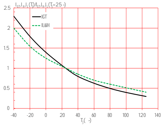
FIG.7: I_{GT}/I_{GT}(T)/I_{GT}(T=25^\circ C) I_{L&H}/I_{L&H}(T)/I_{L&H}(T=25^\circ C)
